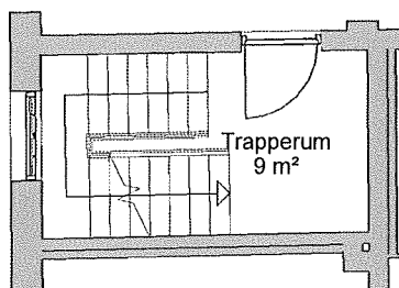
Stueplan - 1:100
